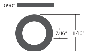
700764 (2.38mm x 11.11mm x 17.46mm)
